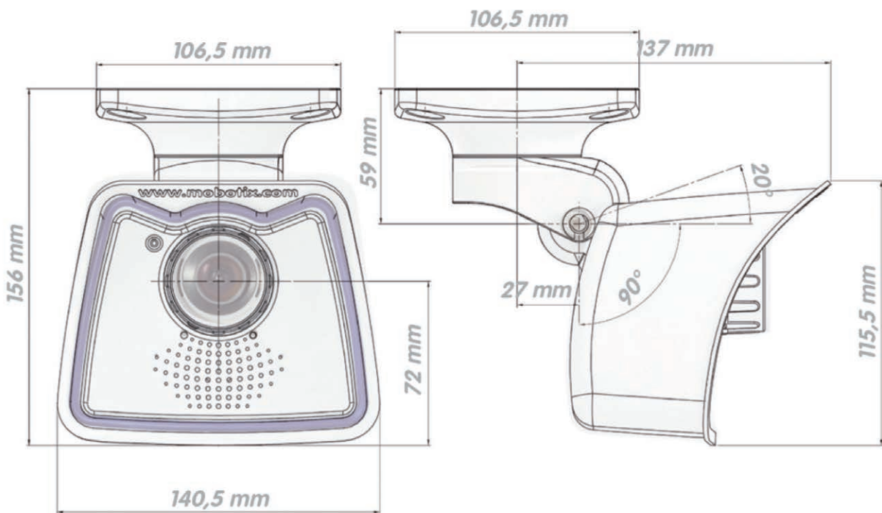
寸法 mm
