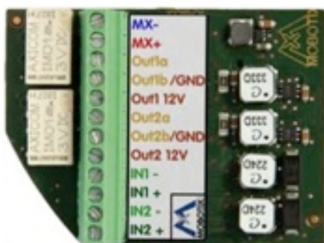
左：外部デバイスに接続する為の緑のターミナルコネクタ付いた MX-Bus-IO-Module の表側
