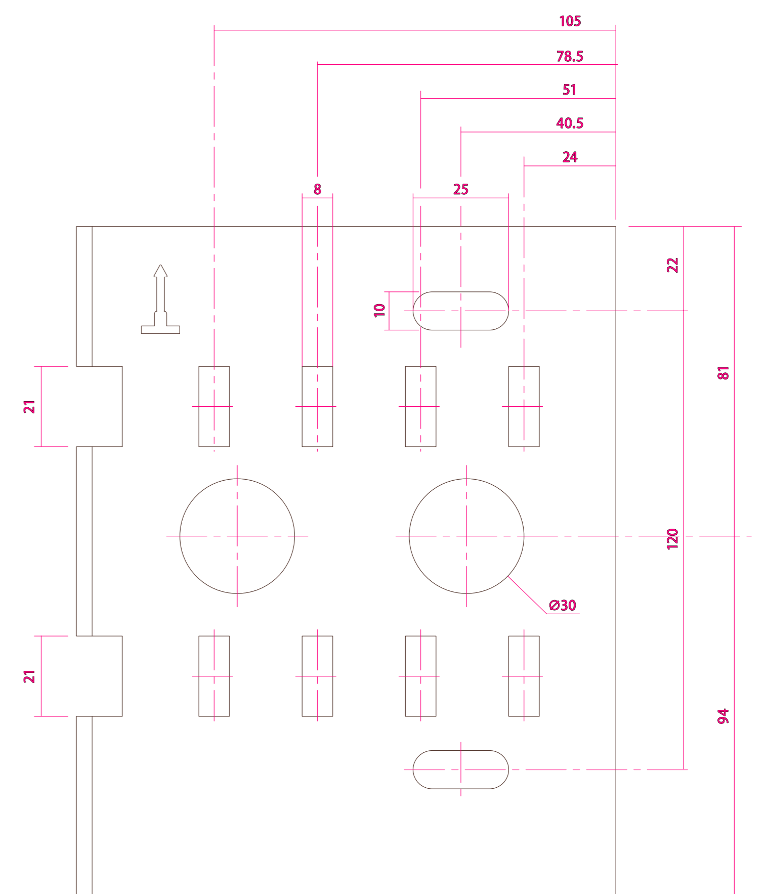
矢视图
